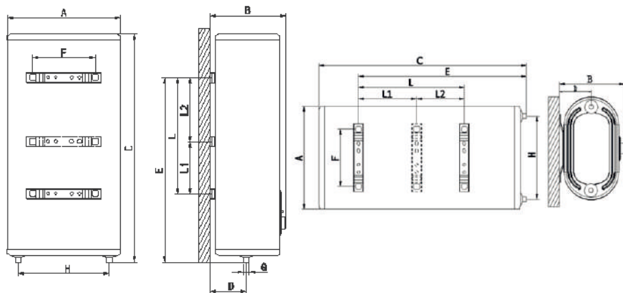
Вертикальная установка
