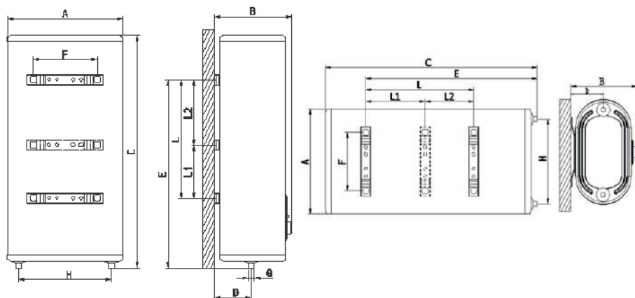
Тік қондырғы
