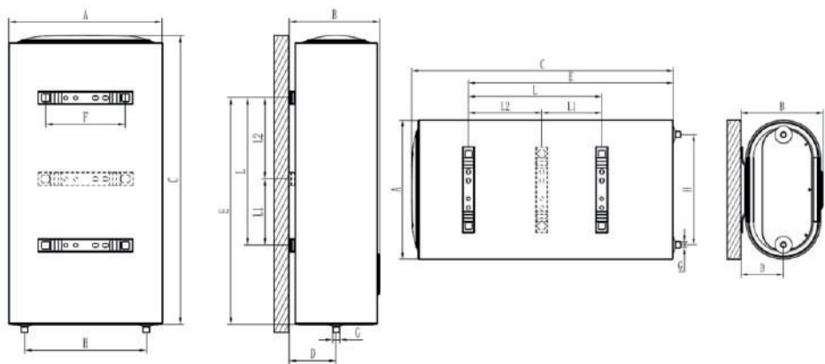
Вертикальная установка
