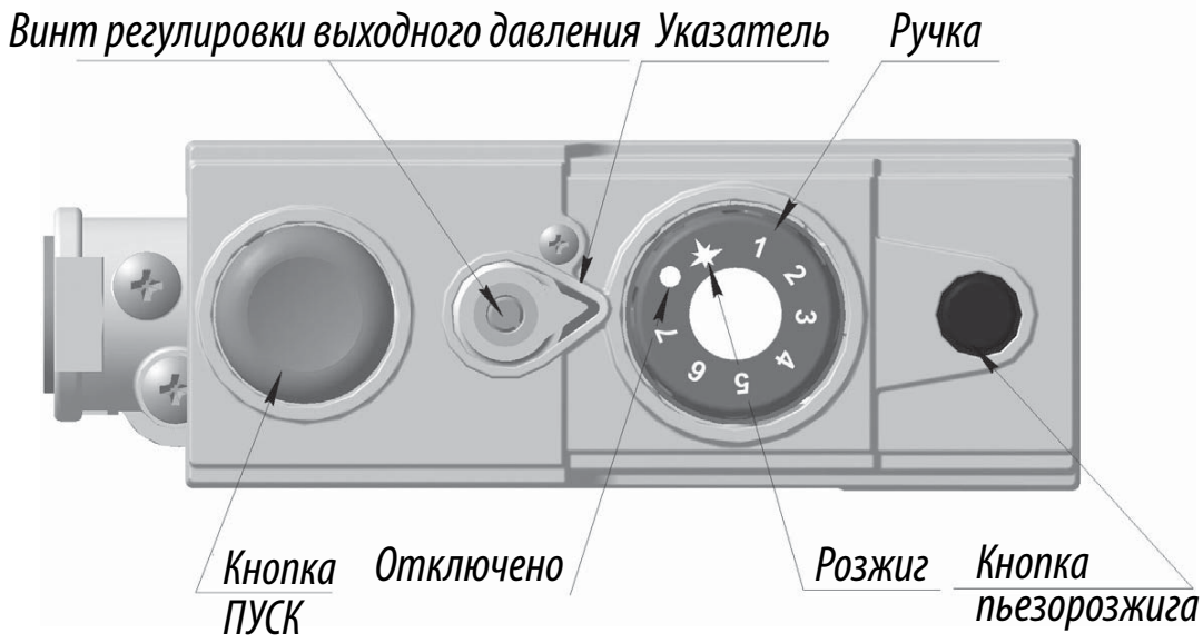
Рисунок 9. Элементы управления на газовом блоке автоматики САБК-АТ
