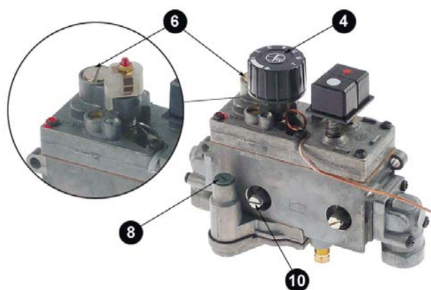
Рисунок 19. Элементы регулировки газового клапана SIT 820 NOVA tv
