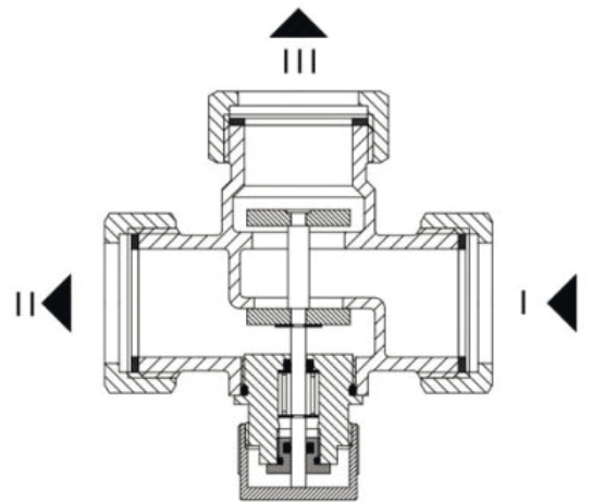
Устройство автоматического трехходового клапана
