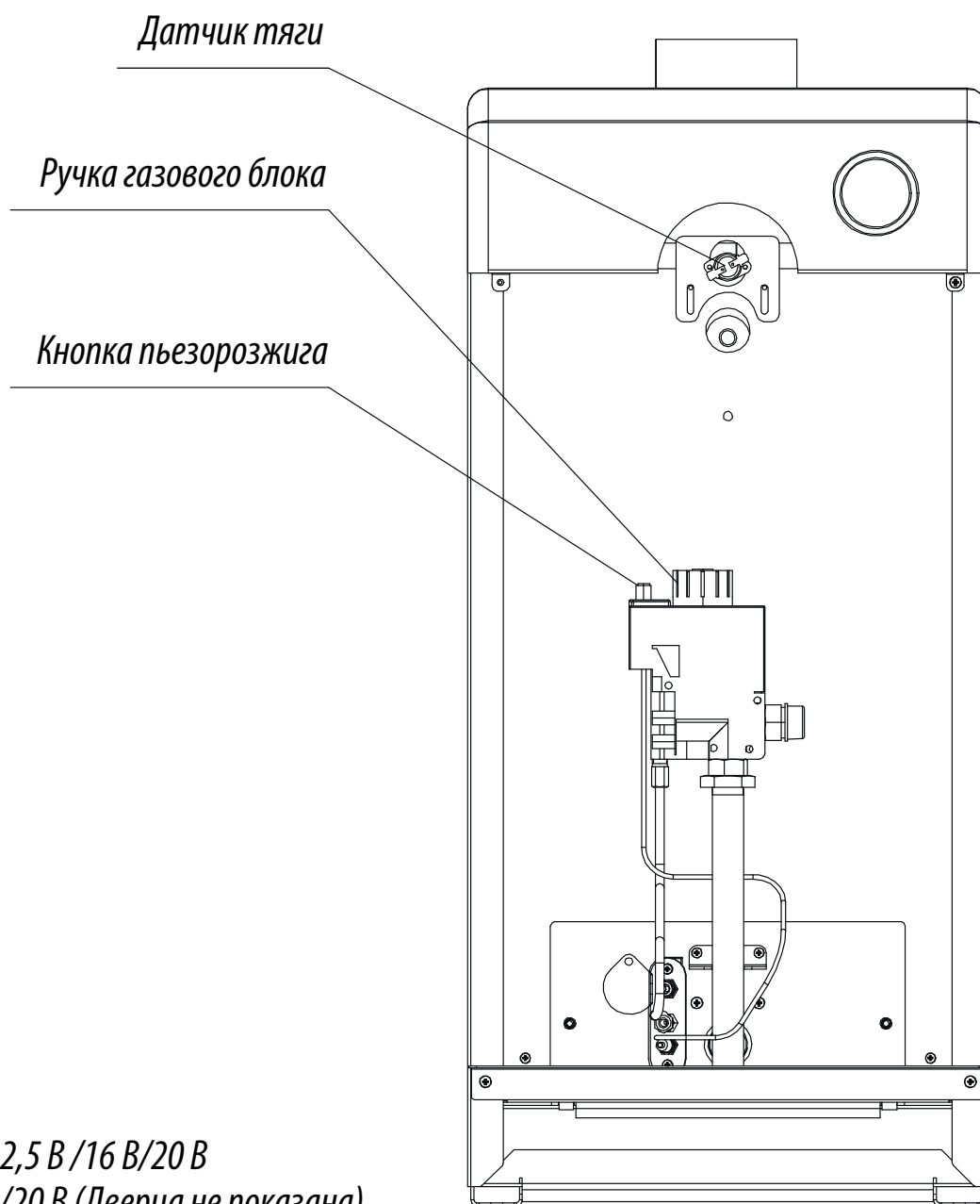
Рисунок 2. Особенности котлов КСГ(КСГВ) с газовым блоком 630 EUROSIT и TGV-307
