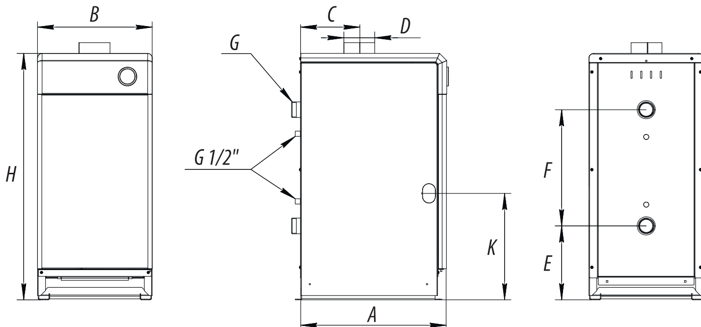
Рисунок 1 - Общий вид, габаритные и присоединительные размеры котлов КСГ (КСГВ)
