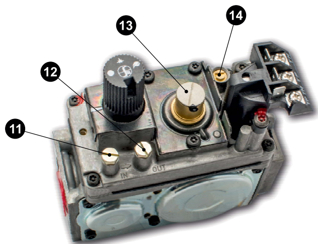
Рисунок 19. Элементы регулировки газового клапана SIT 820 NOVA tv
