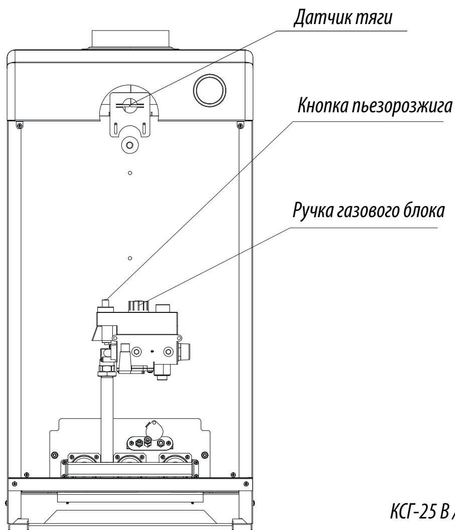
Рисунок 5. Элементы управления на газовом блоке 710 MINISIT
