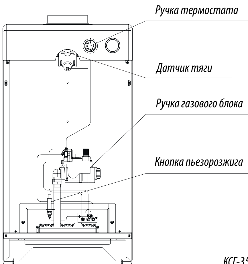
Рисунок 6. Особенности котлов КСГ с газовым блоком SIT 820 NOVA mv
