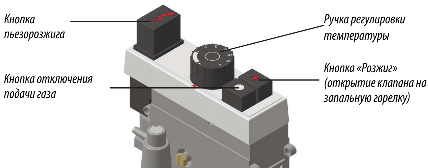
Рисунок 5. Элементы управления на газовом блоке 710 MINISIT
