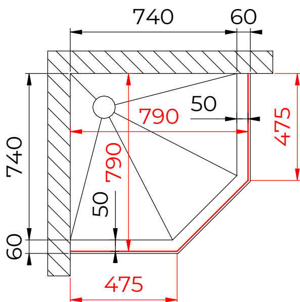
Схема подиума для SV-82 800x800
