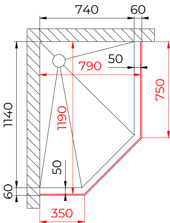
Схема подиума для SV-82 800x1200
