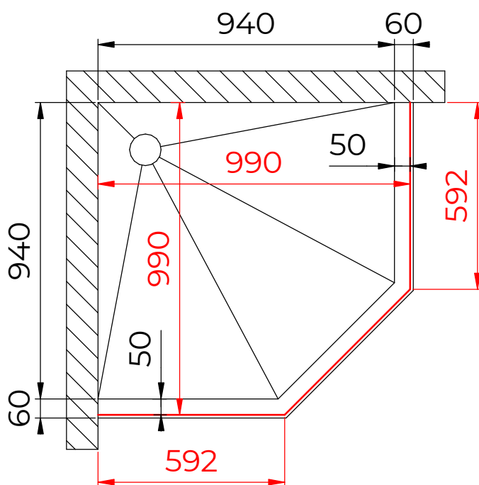
Схема подиума для SV-82 1000x1000
