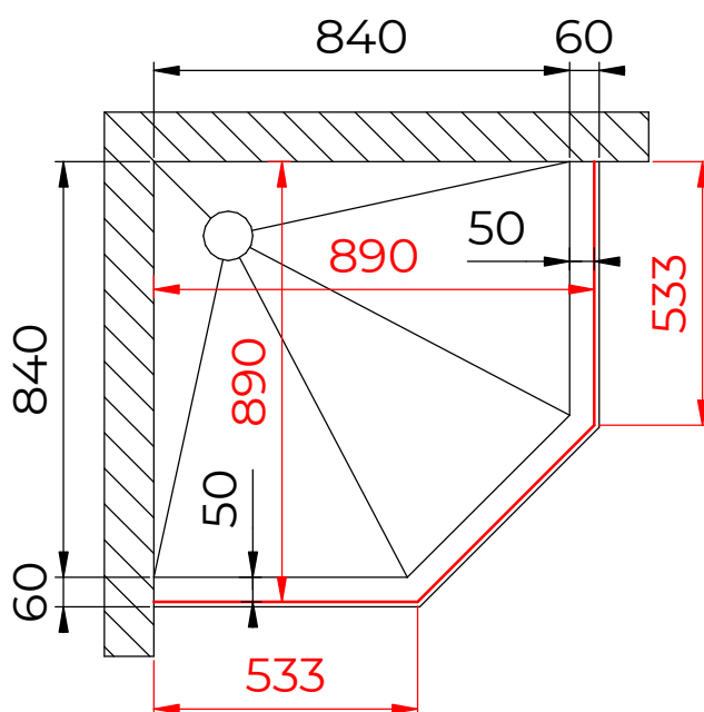
Схема подиума для SV-82 900x900
