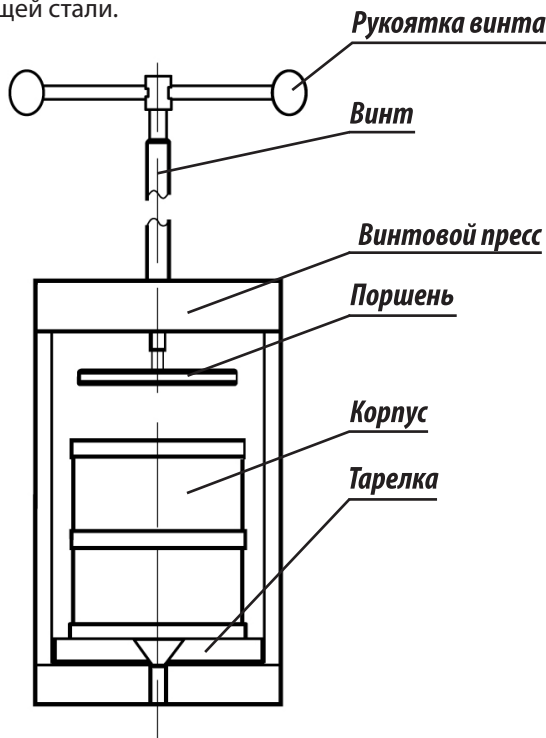
Рис. 1 Устройство изделия
