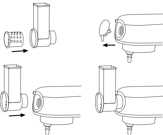
Порядок сборки овощерезки
