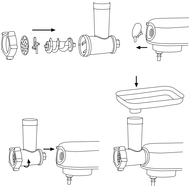
Порядок сборки мясорубки
