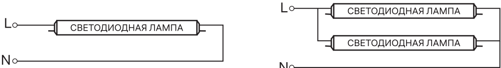
Схема электрическая
