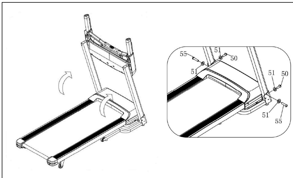
Рисунок 2 — Установка стоек беговой дорожки
