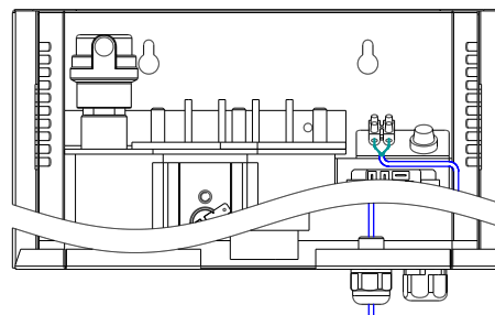
Рис.3 Подключение внешнего термостата
