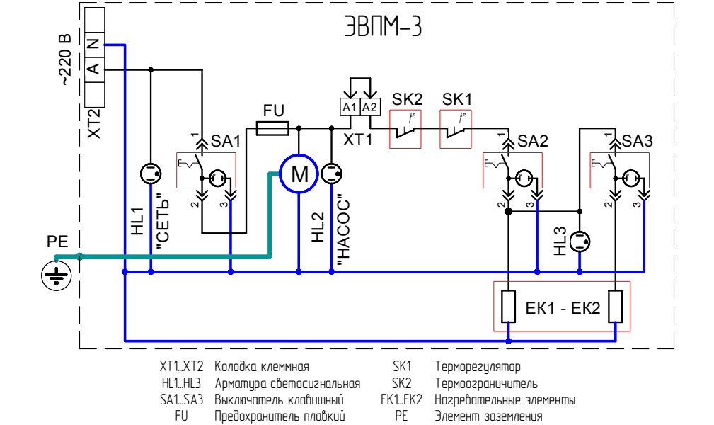
Рис.6.1 Схема электрическая принципиальная ЭВПМ-3
