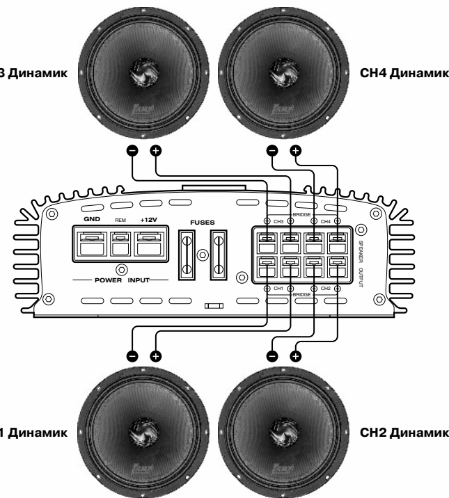
4 канальный усилитель
