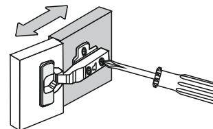
Фронтальная регулировка
