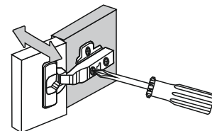
Горизонтальная регулировка
