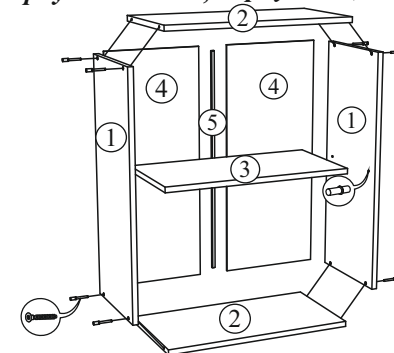
Корпус 1B8/1B8C
