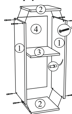
Корпус 1B3
