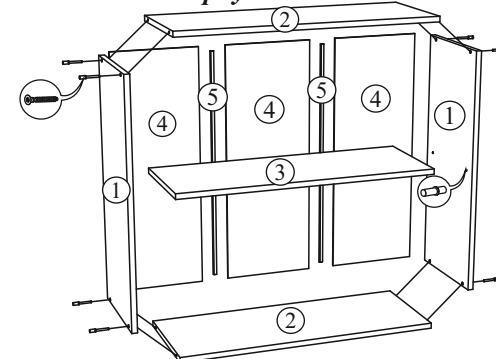
Корпус 1B8/1B8C
