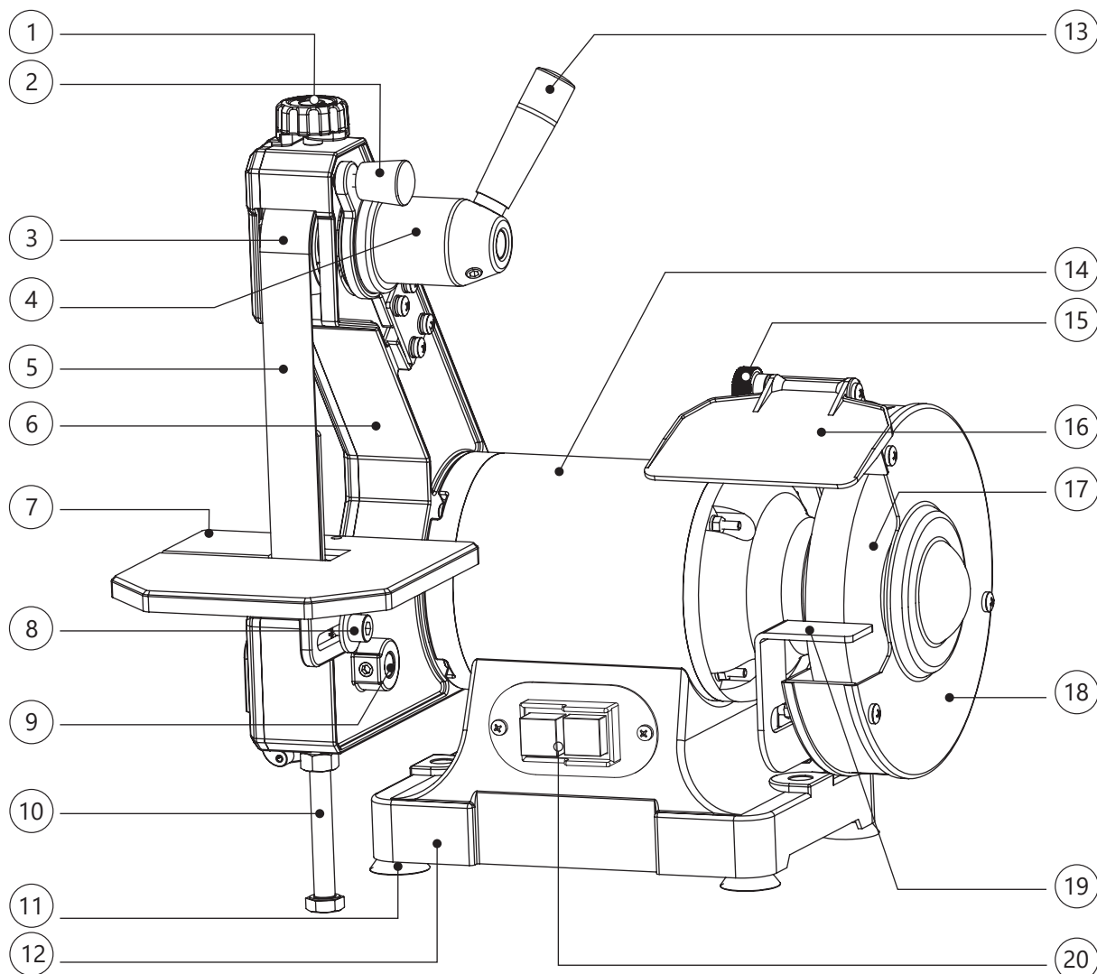
Рисунок 1. Основные элементы станка BELMASH MBG-150/25L.
