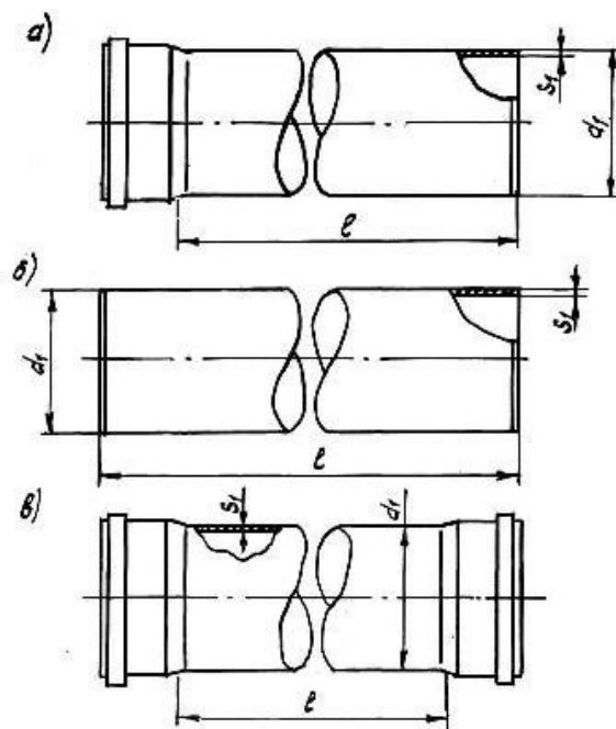
Рисунок 1. Трубы.
