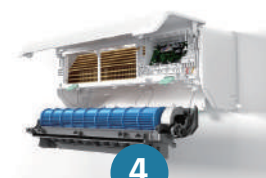
4 Открутите задние фиксаторы извлеките вентилятор и двигатель в сборе
