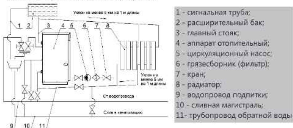
Рисунок 14 – Рекомендуемая гидравлическая схема системы отопления с циркуляционным насосом и схема горячего водоснабжения (ГВС).
