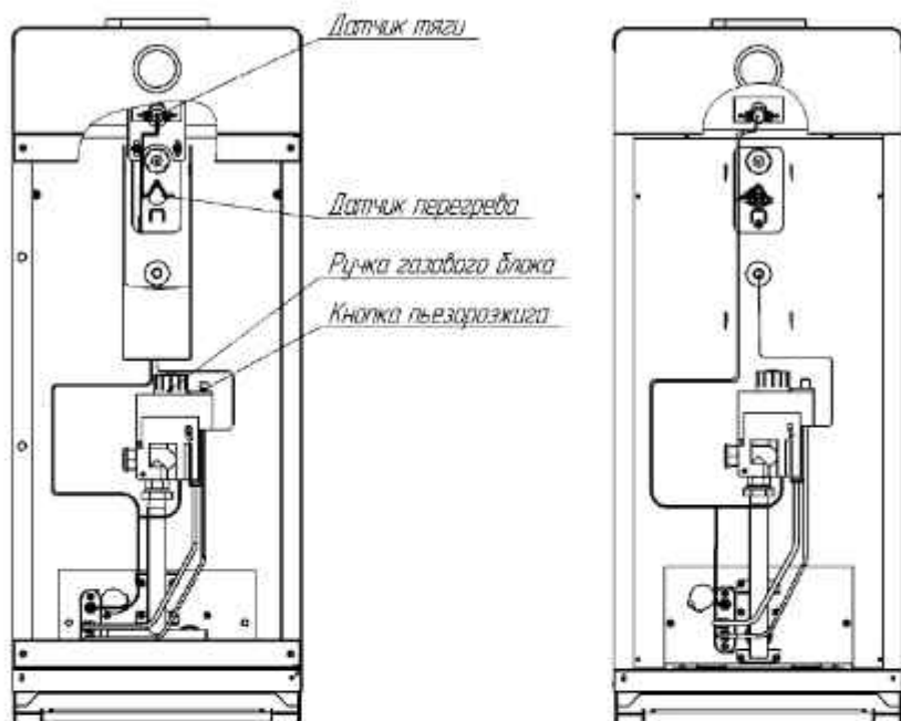
Рисунок 6 - Особенности аппарата с газовым блоком 630 EUROSIT.
