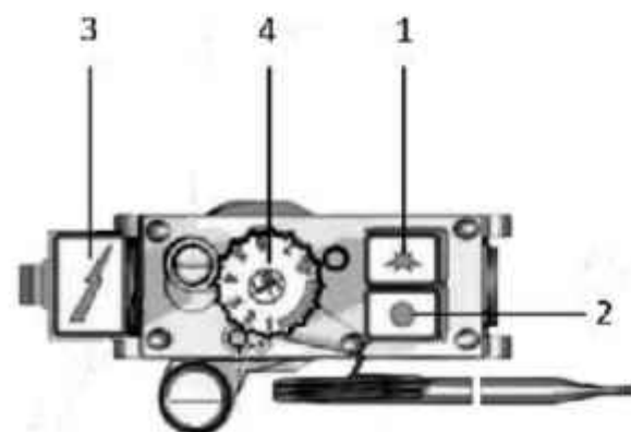
Рисунок 9. Элементы управления на газовом блоке 710 MINISIT.
