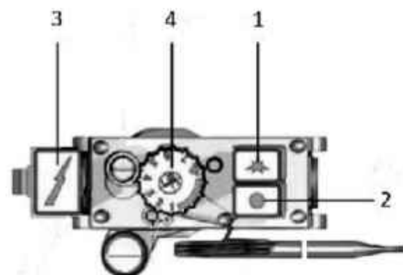
Рисунок 9. Элементы управления на газовом блоке 710 MINISIT.
