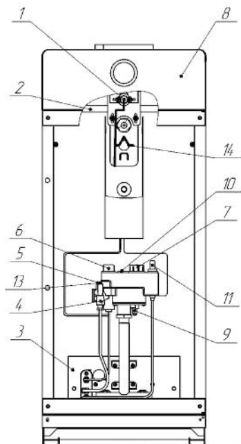
Рисунок 2 - Устройство аппарата с газовым блоком автоматики САБК-АТ.
