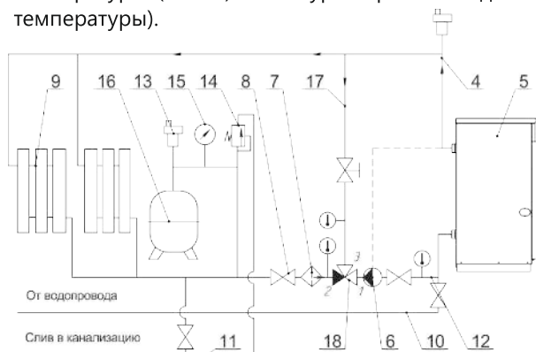
Позиции штуцеров автоматического трехходового клапана:
