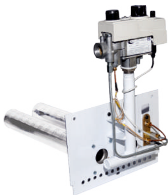
Газовый тракт с блоком САБК-АТ
