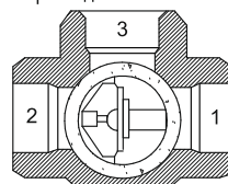
Позиции штуцеров автоматического трехходового клапана:
