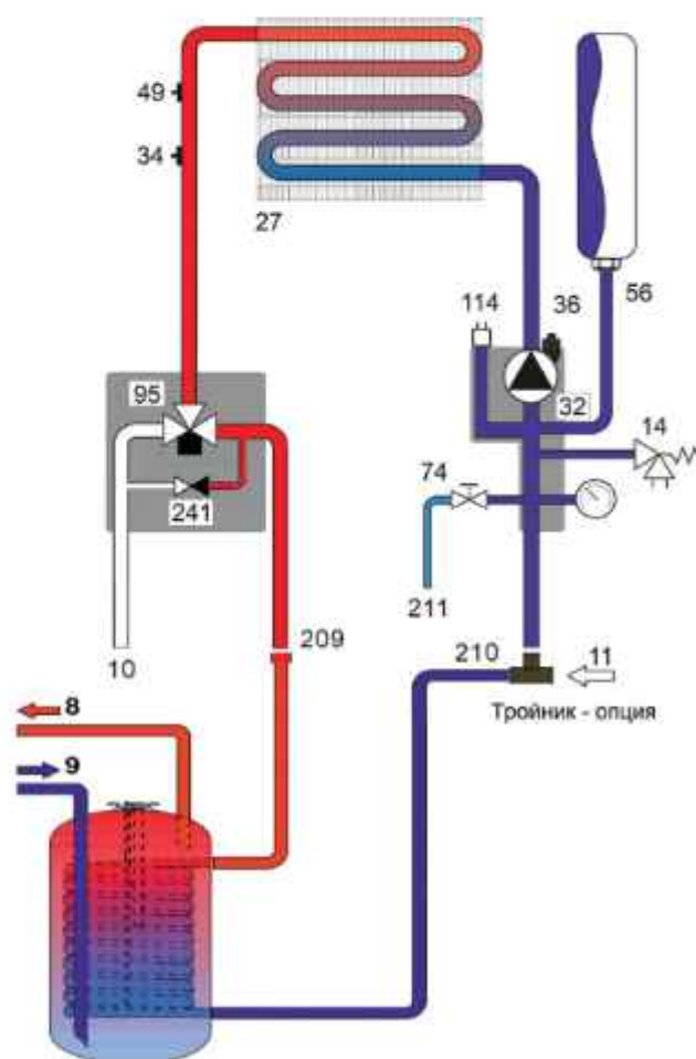
Рис. 19. Схема подключения внешнего бойлера
