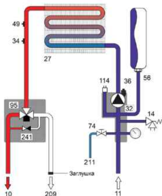
Рис. 18. Отопительный контур
