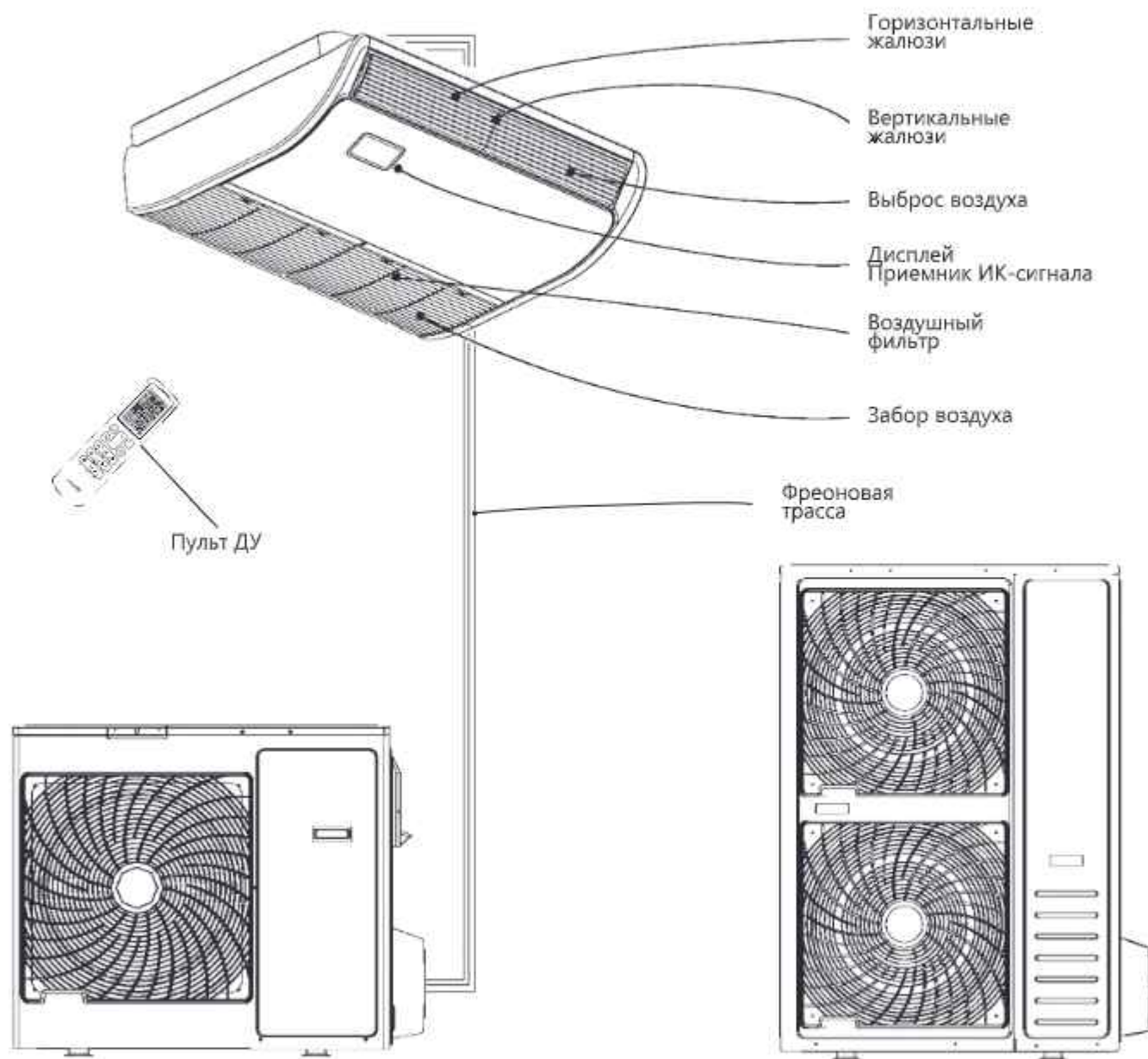
Наружный блок (типоразмер 24/36)
