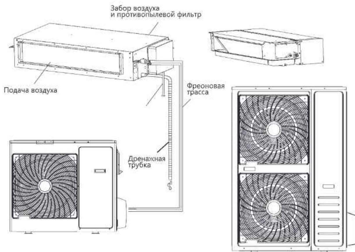
Наружный блок (типоразмер 9/12/18/24/36)
