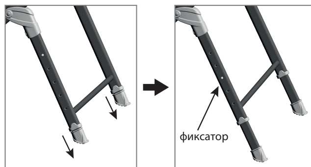
Рис. 2.1 Схема регулировки высоты стола
