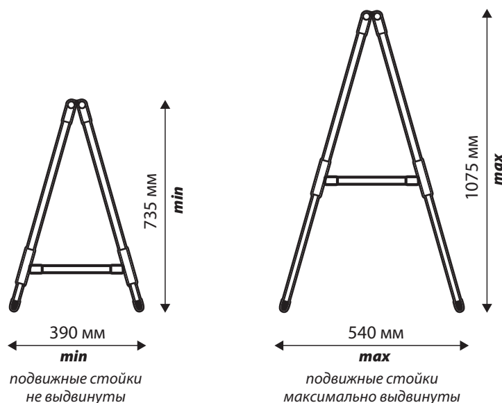
Рис. 2 Размеры мольберта
