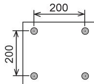
Рисунок 4 – Размеры для выбора настенного кронштейна
