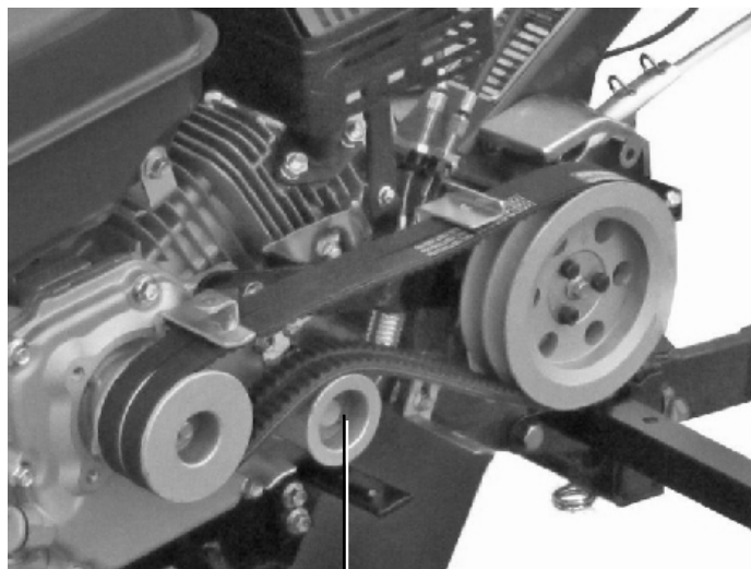
Шкив натяжной
