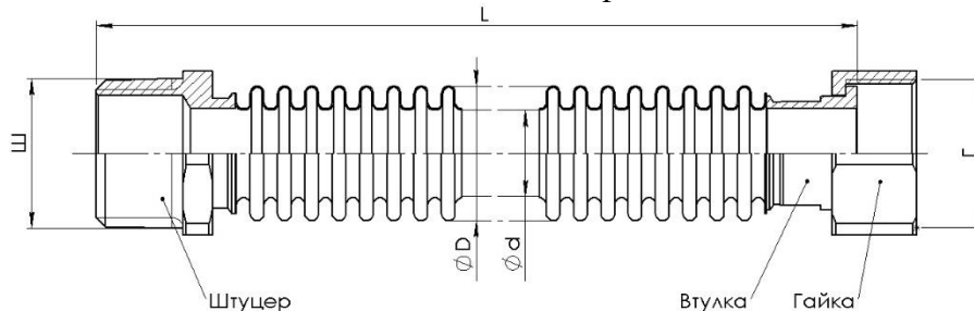
Рис.1. Шланг газовый сильфонного типа.
