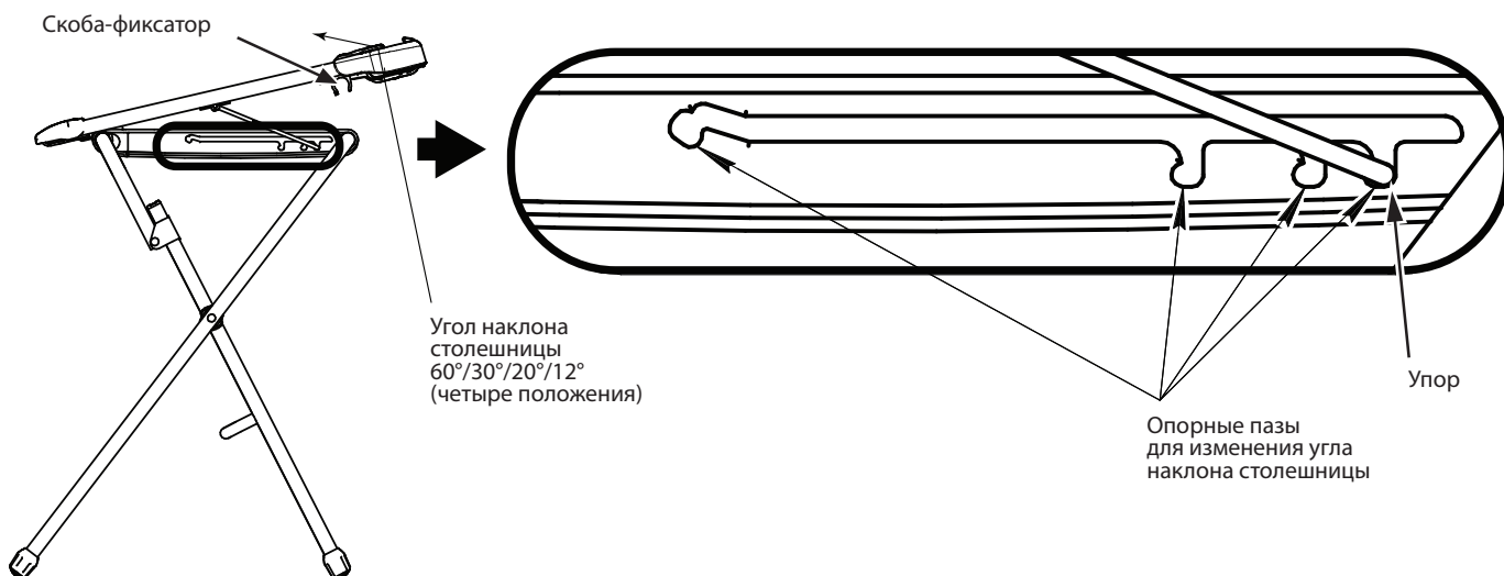
Рис. 3 Схема изменения наклона столешницы
