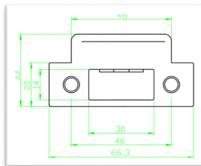
Рис. 2 Ответная планка
