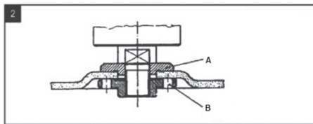
(А- прижимный фланец, В – зажимная гайка)
