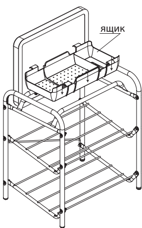
Рис 3. Установка ящика
