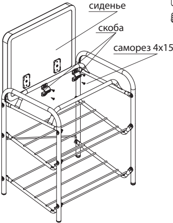
Рис 2. Сборка сиденья
