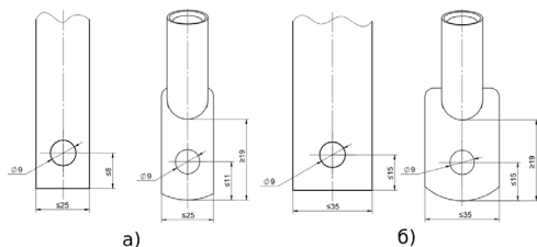
Рисунок 5 - Форма и размеры присоединяемой шины максимального сечения
