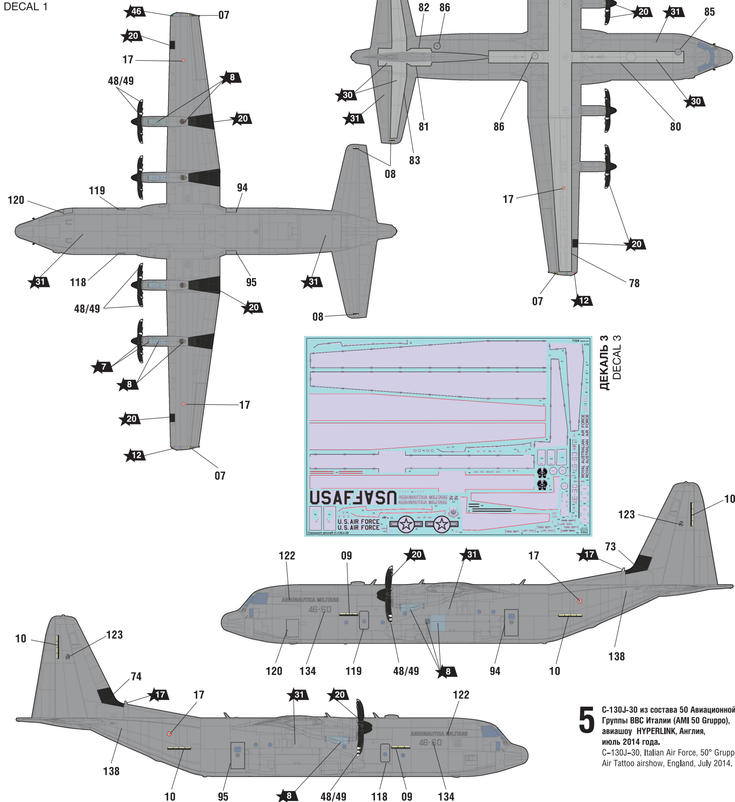
ДЕКАЛЬ 1 DECAL 1
