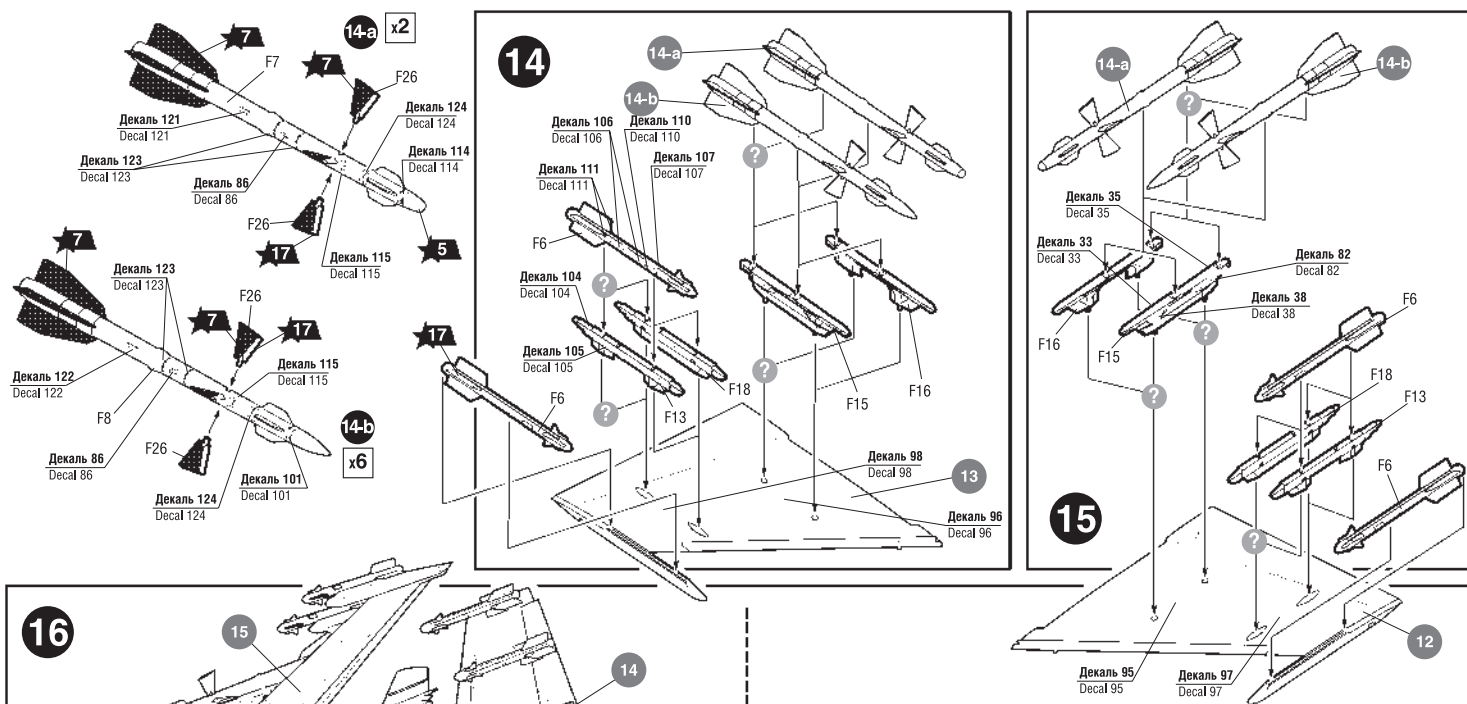
ВАРИАНТЫ СБОРКИ 1, 2 ASSEMBLING VERSIONS 1, 2
