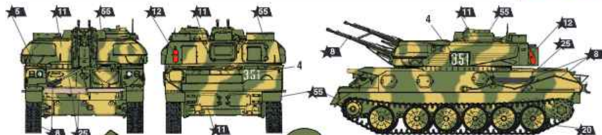
ЗСУ-23-4 из состава армии СССР, Афганистан, Алхейль, лето 1987 г. ZSU-23-4 Soviet Armed Forces, Afghanistan, Alkheil, summer 1987
