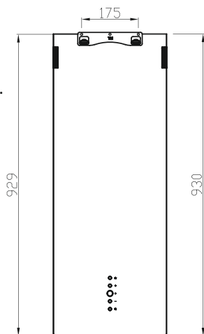
Рис. 8 Схема монтажа вытяжки
