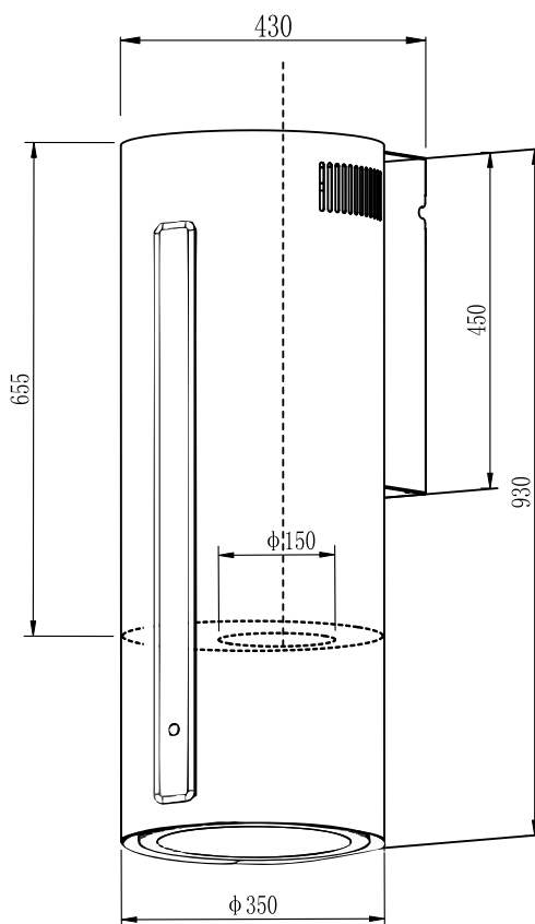
Рис. 1 Внешний вид кухонной вытяжки и схема размеров
