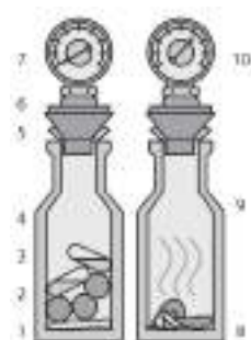
Рис. 10. Прибор СМ (измерение при помощи карбидно-кальцевого метода)
