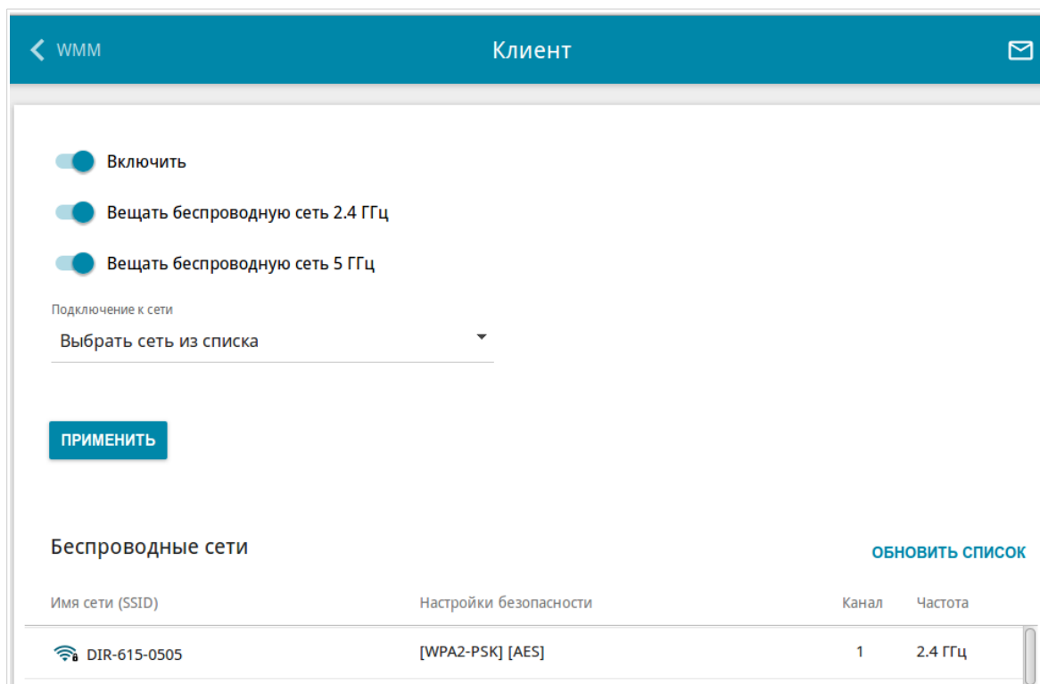
Рисунок 91. Страница для настройки маршрутизатора в качестве клиента.
