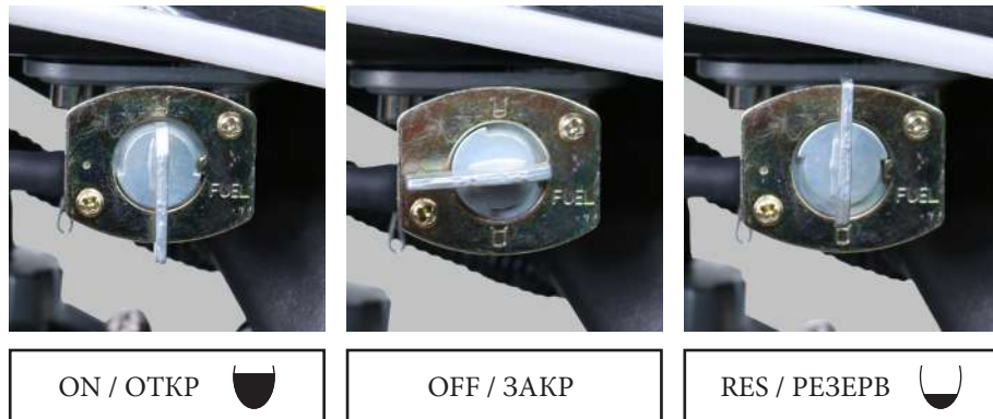
Фото 3.1. Положения крана подачи топлива.
