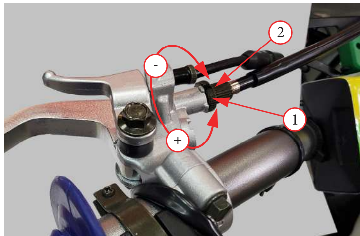
Фото 5.12. Регулировка свободного хода рычага сцепления.
