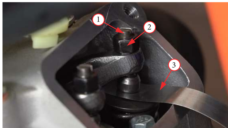
Фото 5.40. Регулировка теплового зазора: 1 – регулировочный винт; 2 – контргайка; 3 – щуп.
