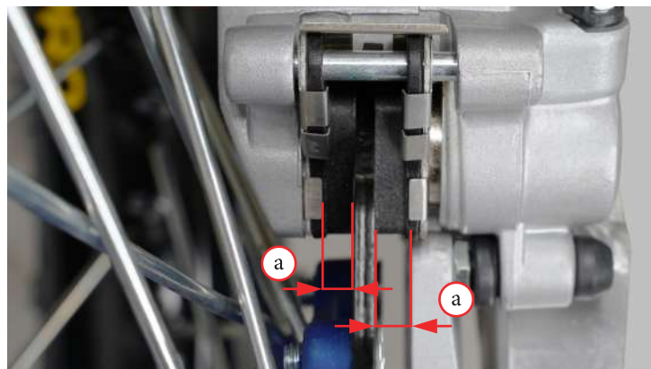
Фото 5.21. Контроль тормозных колодок.
