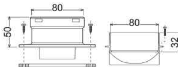
рис. 30 - Соединительный элемент для отдельных труб
