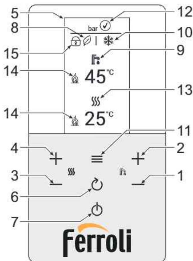
Рис. 1- Панель управления
