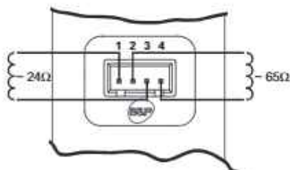
Рис. 30 - Электрический разъем для подключения газового клапана
