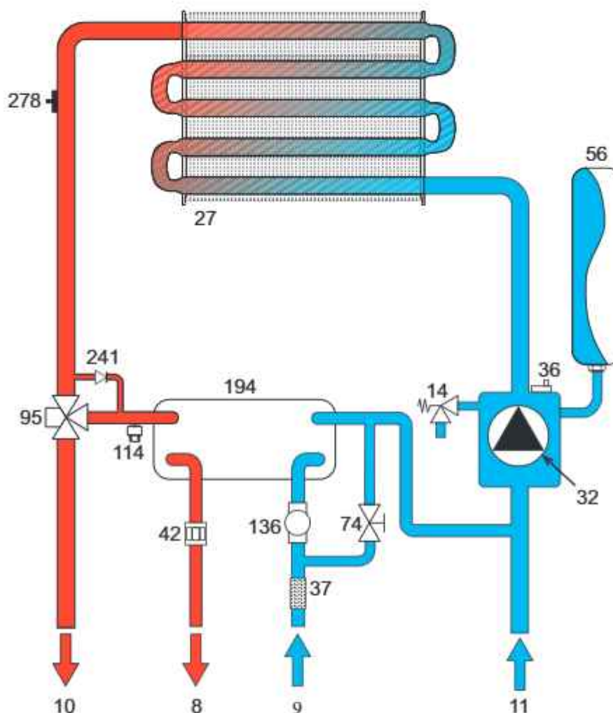
Рис. 36- Гидравлическая схема
