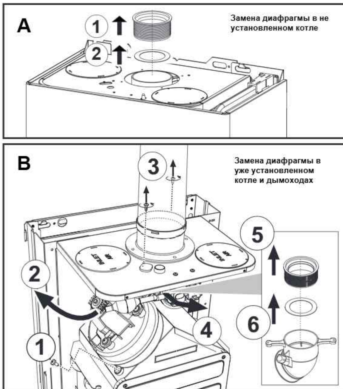
рис. 26- Замена диафрагмы
