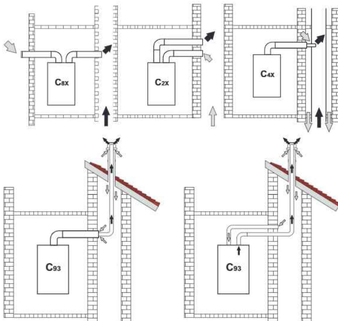
рис. 31 - Примеры подсоединения к дымоходам (⇨ = Воздух / ⇨ = Дымовые газы)
