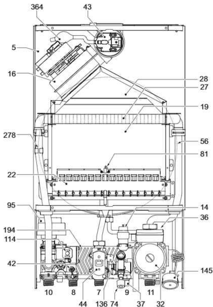
рис. 42- Общий вид - DIVATOP D F
