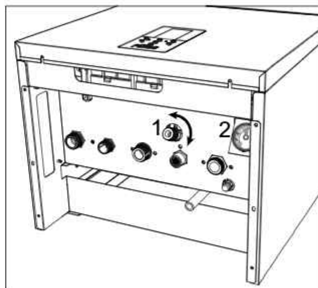
Рис. 24 Ручка крана заполнения системы
