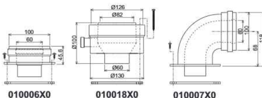
рис. 28- Исходные принадлежности для коаксиальных труб
