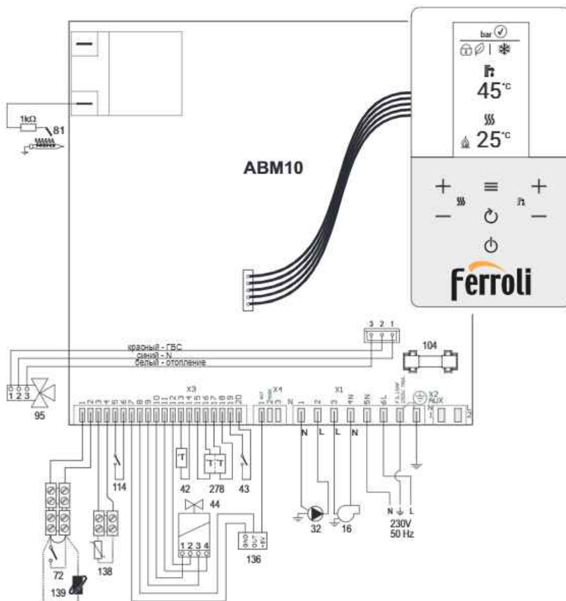
рис. 46- Электрическая схема
