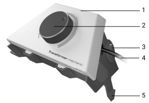
Рис. 1 Блок управления
