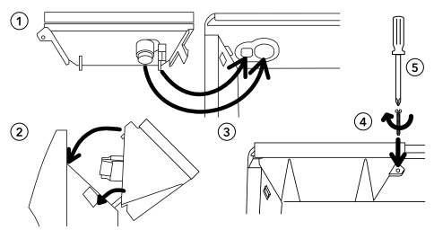
Рис. 3 Схема установки
