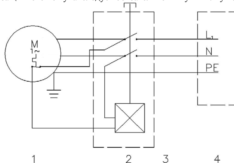
Рис. 2. Электрическая схема бетономешалки BWE-SK-120L/z, BWE-SK-150L/z, BWE-SK-170L/z, BWE-SK-190L/z
