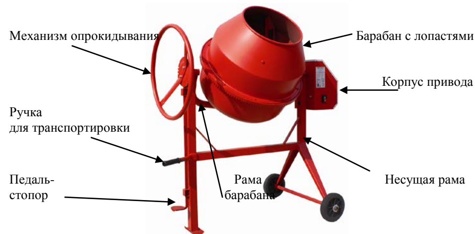
Рис. 1 Электрическая гравитационная бетономешалка BWE-SK-120L/z , BWE-SK-150L/z , BWE-SK-170L/z , BWE-SK-190L/z
