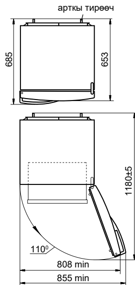
2-сүрөт – Муздаткыч (үстүнөн көрүнүшү)
