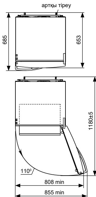
2-сурет – Тоғазытқыш (жоғарыдан қарағандағы түрі)
