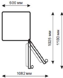
Uskunaning ishchi o'lchamlari
