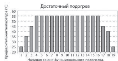
Рис. 16. Достаточный подогрев
