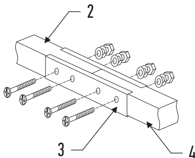
Рис.3 Установка узла согласования на основной траверсе
