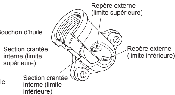
Fig. 2 Tuyau d'huile
