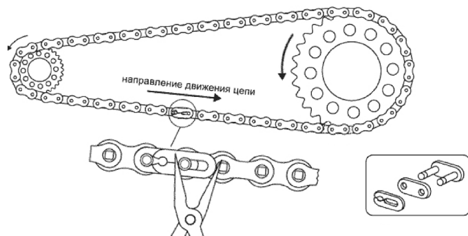
Рисунок 5.31. Установка элементов замка цепи
