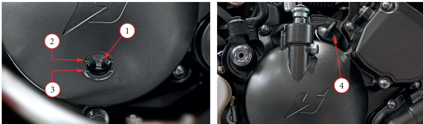
Фото 5.1.1. Исполнение смотрового окна и крышки горловины двигателей
