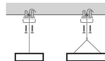
Рис. 4 Схема подвешного монтажа светильника PSO-01
