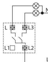
Рисунок 2. Схема подключения двухклавишного выключателя.
