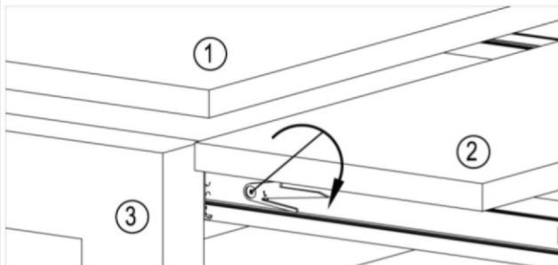
СХЕМА РЕГУЛИРОВКИ УРОВНЯ ВЫДВИЖНОЙ СТОЛЕШНИЦЫ
