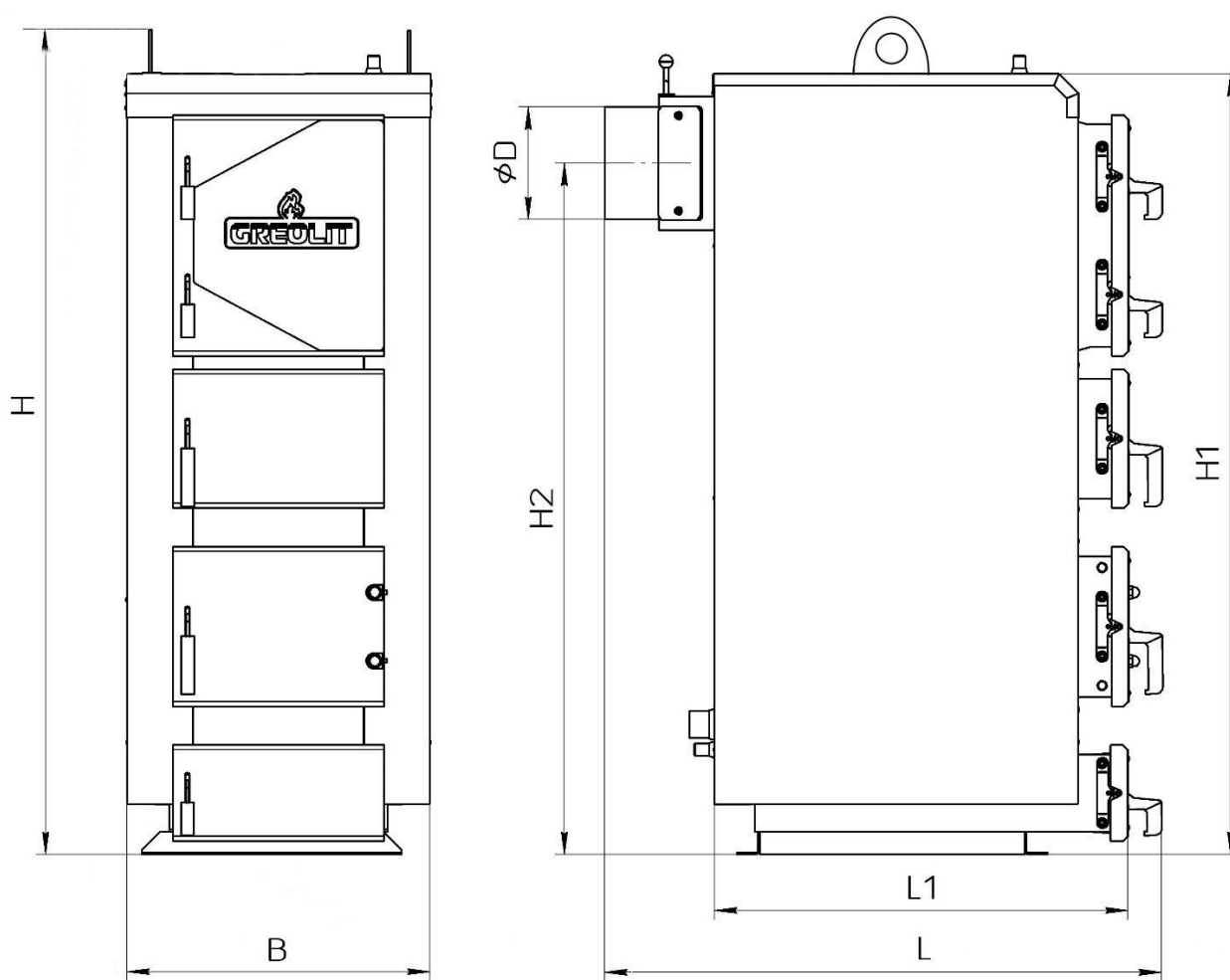
Рисунок 1 - Габаритный чертёж котла типа GREOLIT PROFi (50-99кВт)
